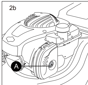
2b Press the primer bulb (A) 3-5 times.
